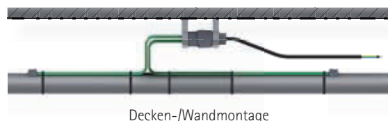
Decken-/Wandmontage
