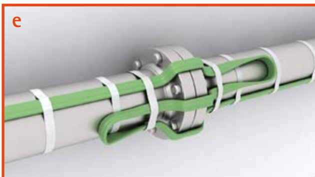
Verlegung an Flanschen
